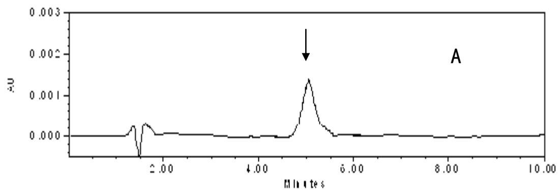
图 A1 常山酮标准溶液色谱图 (100 ng/mL)
